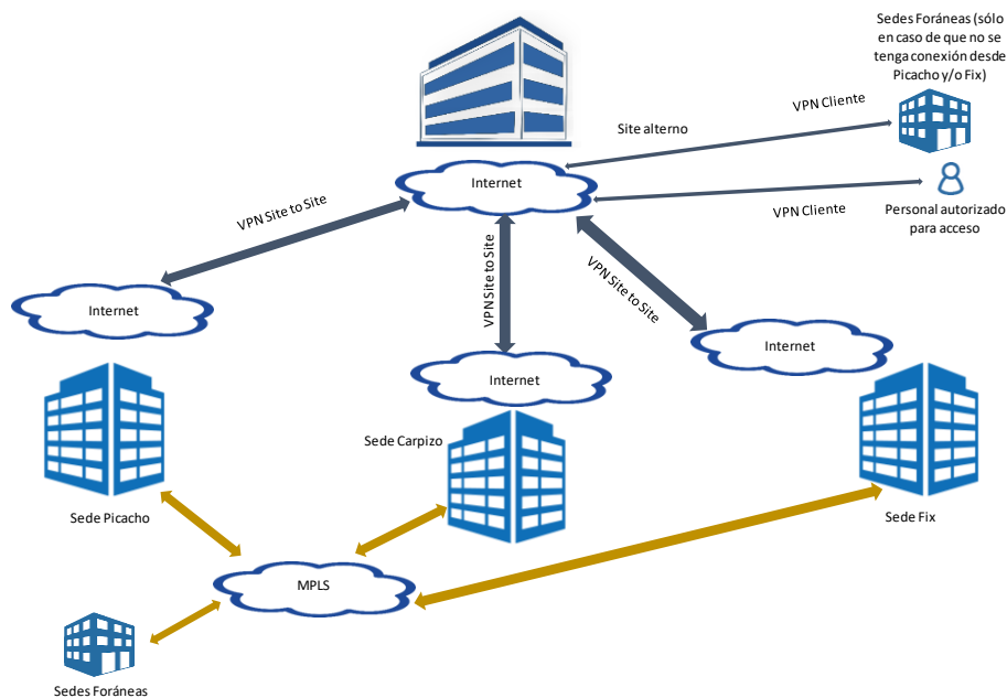
Figura 2. Esquema de conectividad
